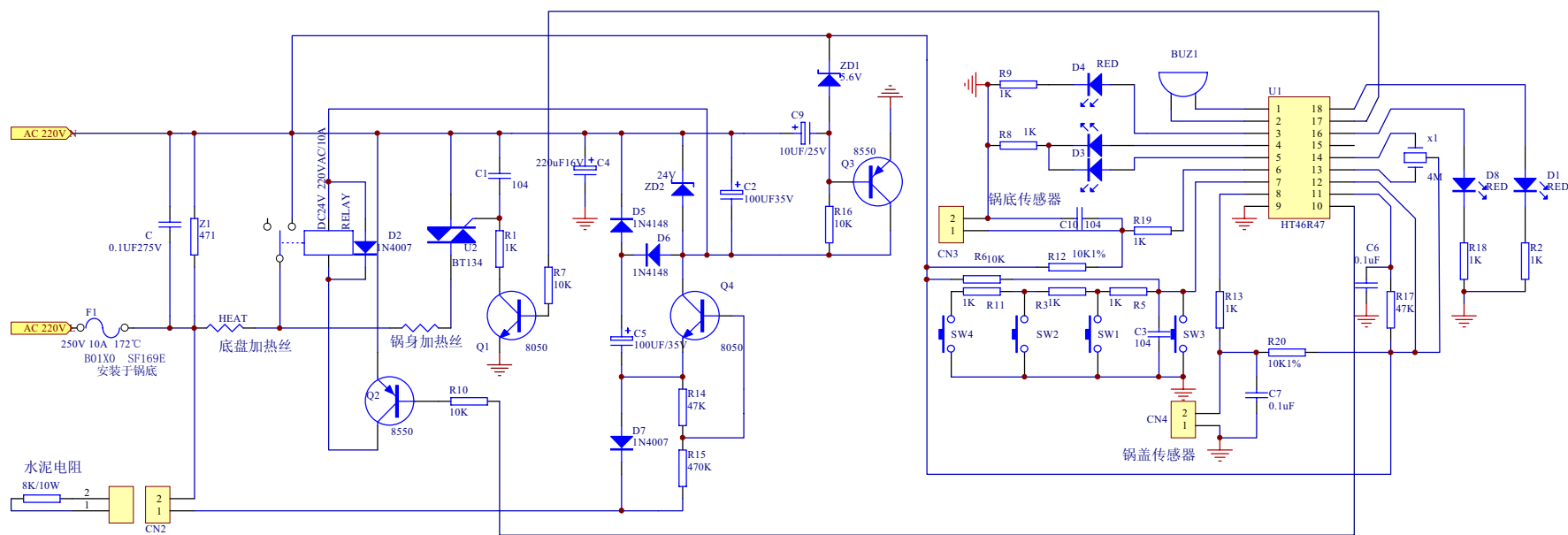
16YD2控制板
