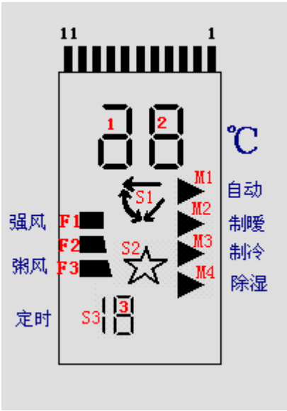
简单空调遥控器 LCD 真值表
